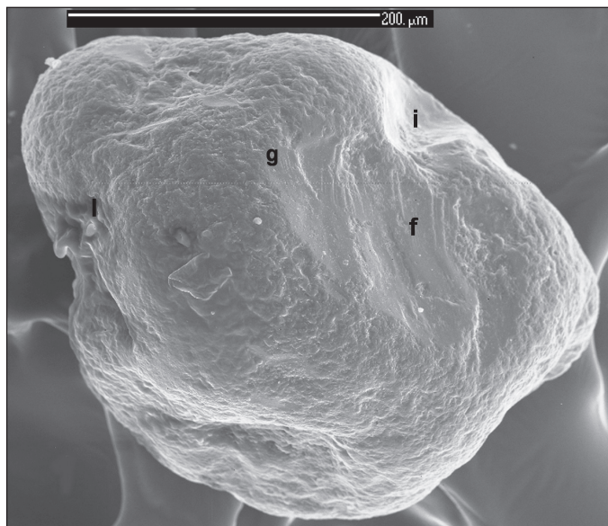
Obr. 1 – Nejčastější tvary vyskytující se na povrchu zrna: f – paralelní rýhy, g – V-jamky, i – rovné brázdy, l – křemičité skrvčky. Vzorek eolického sedimentu; Praha-Klárov.
