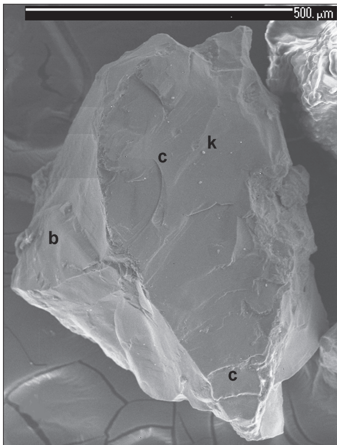
Obr. 4 – Nejčastější tvary vyskytující se na povrchu zrna: b – rovné stupně, c – obloukové stupně, k – přilnavé částice. Vzorek deluvia; údolí Bílého Labe, Krkonoše.
