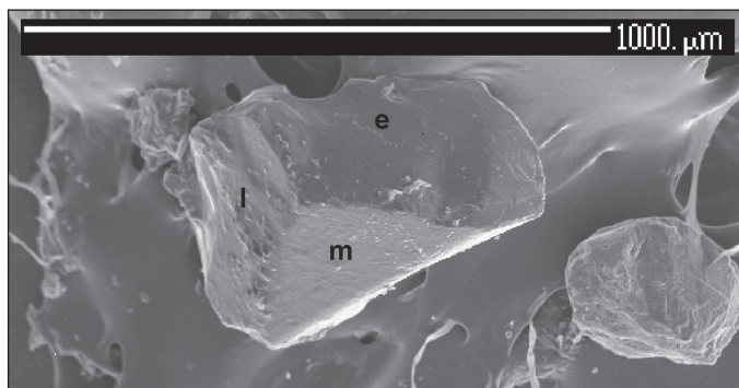
Obr. 3 – Nejčastější tvary vyskytující se na povrchu zrna: e – klikaté hřbítky, l – křemičité skrvčky, m – křemičitý povlak. Vzorek fluvialního sedimentu; údolí Bílého Labe, Krkonoše.
